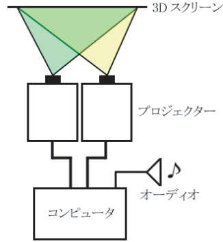
3D静止画上映用システム
