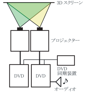
3D動画上映用システム
